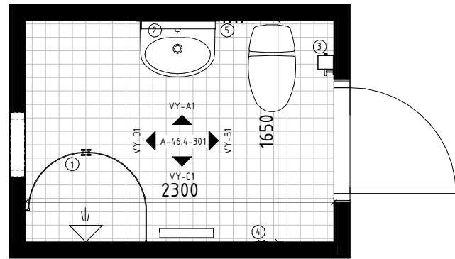
BADRUM TYP 1
