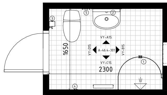
BADRUM TYP 1S
